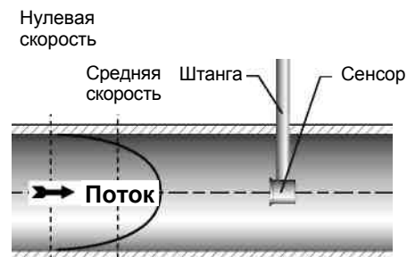
Рис.1.1. Принцип работы. Локальная скорость измеряется на глубине погружения, преобразуется в среднюю скорость потока и затем в средний объемный расход..
