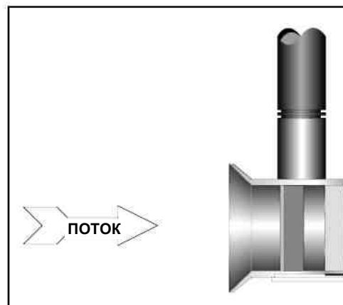
Рис.6.11. Вход сенсора. Когда производится сборка штанги, убедитесь в том, что стрелка направления потока и вход вихревой головки сенсора (рас-труб) направлены навстречу друг другу.
