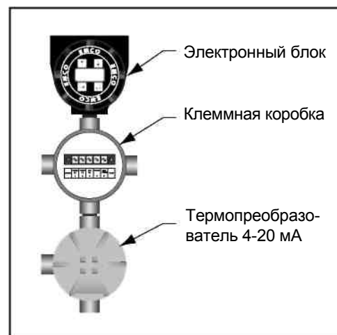
Рис.6.29. Расположение клеммной коробки
