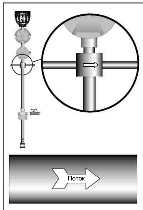
Рис.3.12. Ориентирование V-Bar-700. Направьте рычаги ориентации параллельно оси трубопровода так, чтобы стрелка на корпусе была по направлению потока среды.
