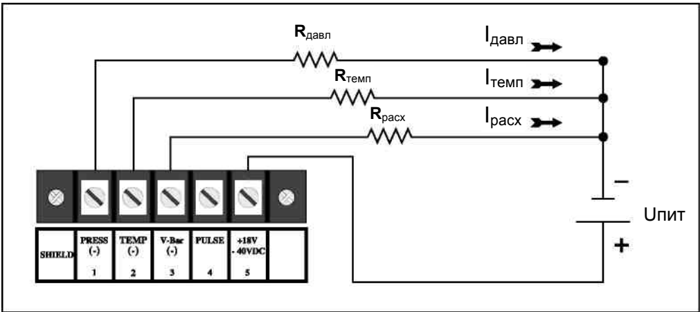
Рис.4.9. Схема подключения аналогового выхода расхода, датчика давления и температуры
