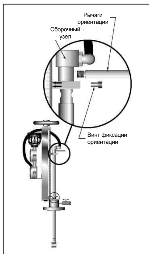
Рис.6.28. Извлечение сенсора V-Bar-900. Отвернуть штангу от монтажного соединения и извлечь штангу вытягиванием со дна расходомера..
