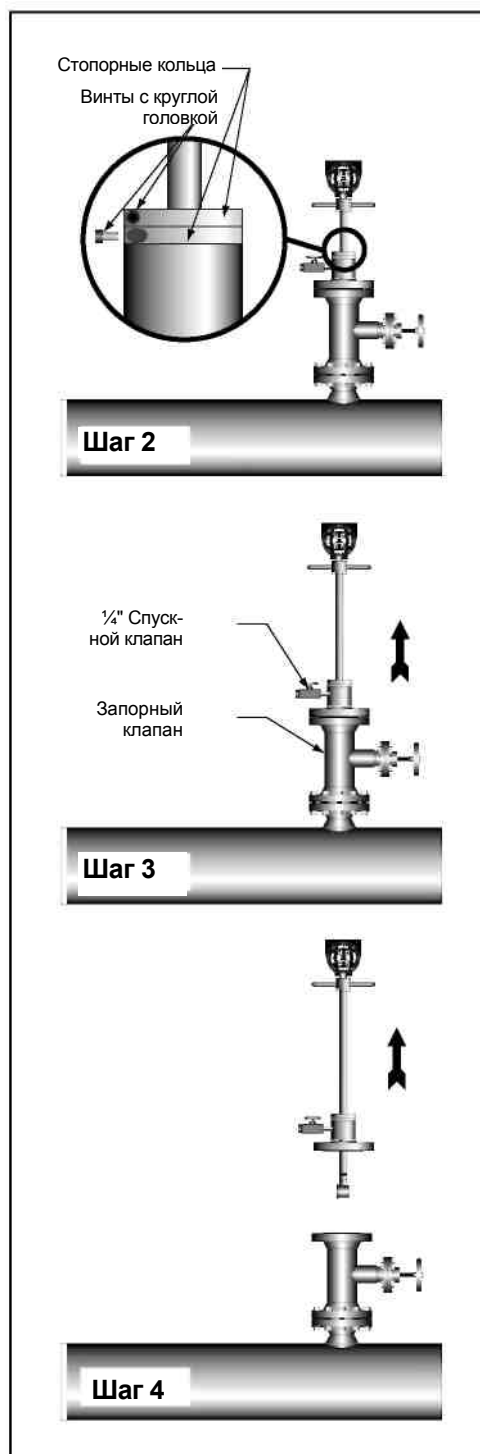
Рис.6.19. Извлечение V-Bar-800/80S
