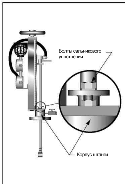
Рис.3.25. Размещение болтов сальникового уплотнения. Чтобы зафиксировать штангу, затяните болты сальникового уплотнения, размещенные на корпусе штанги.
