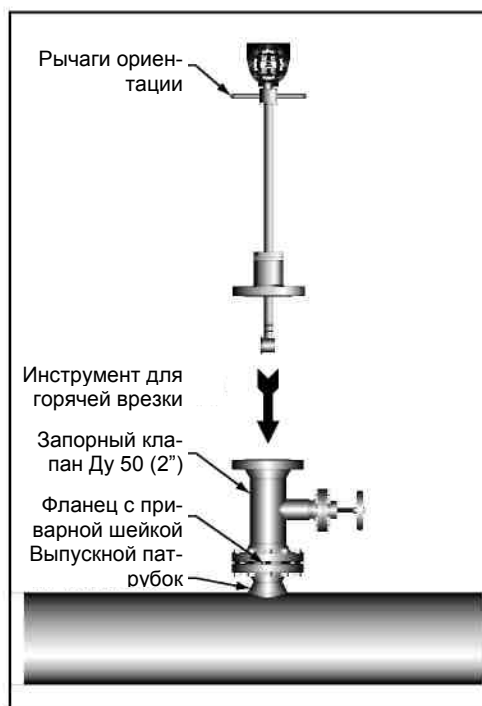
Рис.3.13. Горячая врезка V-Bar-800/80S фланцевого присоединения к трубопроводу
