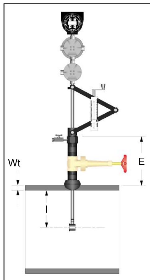
Рис 3.3. Отсчет по шкале V-Bar-600/60S. Отсчет по шкале это цифра на которую указывает курсор. Отсчет по шкале равен глубине погружения сенсора.
