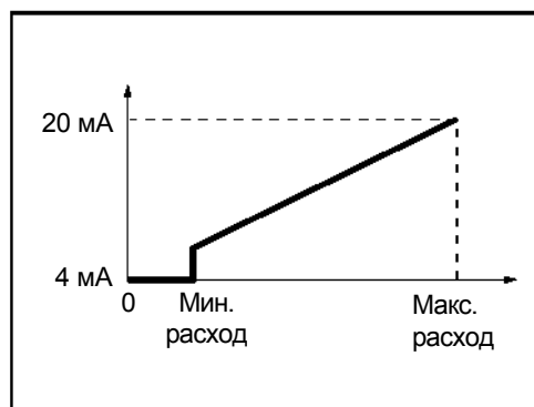
Рис.5.5. Линейный аналоговый выход
