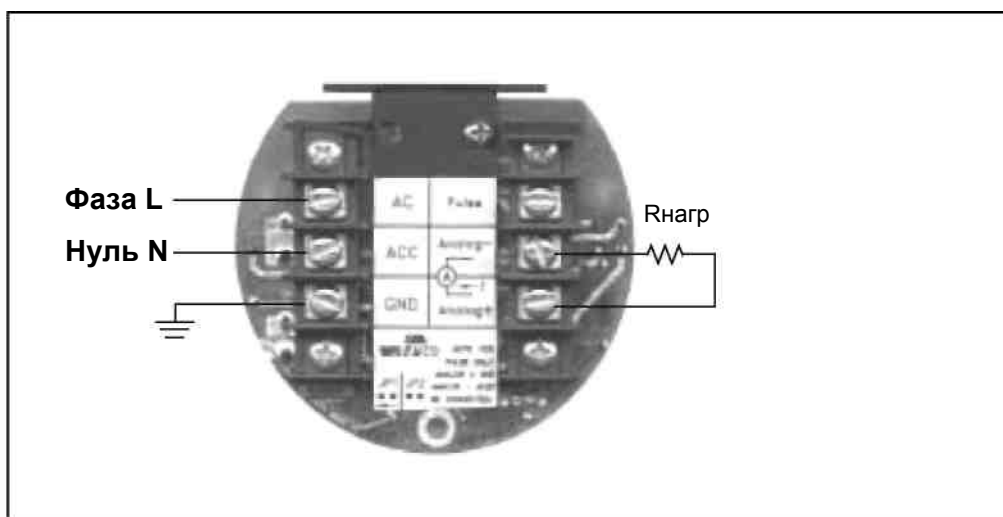
Рис.4.11. Схема подключения с аналоговым выходом
