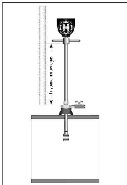
Рис.3.11. Окончательное позиционирование V-Bar-700. Вручную введите штангу в трубу до вычисленной глубины.
