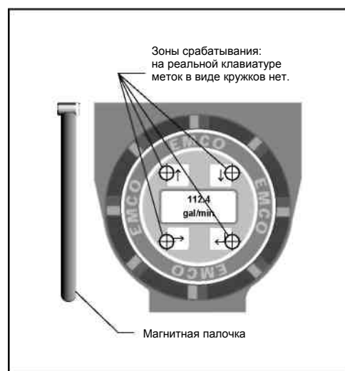
Рис.5.2. Бесконтактное управление клавиатурой. Для «нажатия» клавиши поместите магнитную палочку в отмеченную зону и быстро уберите ее.
