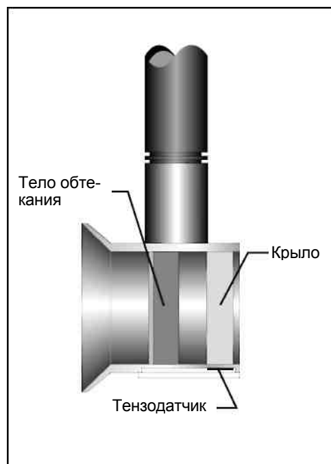
Рис.1.2. Поперечное сечение первичного преобразователя расхода (сенсора) V-Bar.
