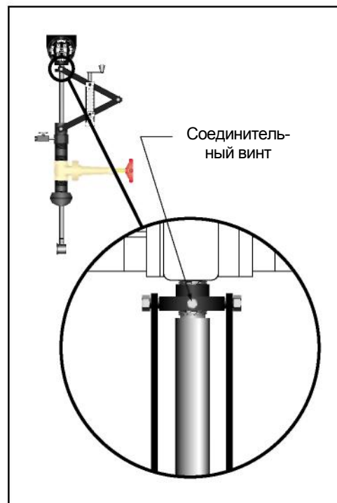
Рис.6.7. Расположение соединительного винта
