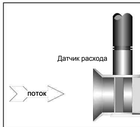
Рис.6.23. Вход вихревой головки сенсора. При сборке штанги стрелка направления потока и вход вихревой головки сенсора (раструб) направлены навстречу друг другу.
