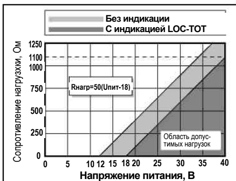
Рис.4.4. График нагрузок для аналогового выхода
