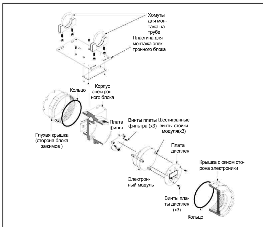
Рис.6.2. Электронный блок раздельного исполнения
