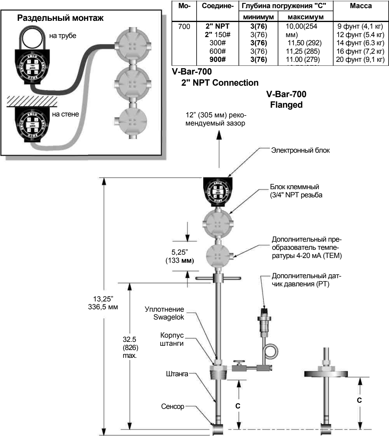
Рис.6-16. Габаритные размеры V-Bar-700. Все размеры в дюймах и миллиметрах
