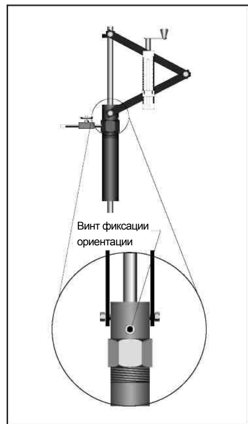
Рис.3.6. Расположение винта фиксации направления. Чтобы зафиксировать штангу в нужном положении, затяните винт фиксации ориентации.
