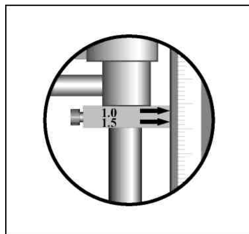
Рис.3.24. Отсчет по шкале V-Bar-910/960. Отсчет по шкале производится против стрелки указателя 1.0↑ и равен глубине погружения сенсора.
