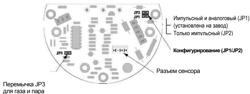
Рис.4.1. Плата фильтра V-Bar™
