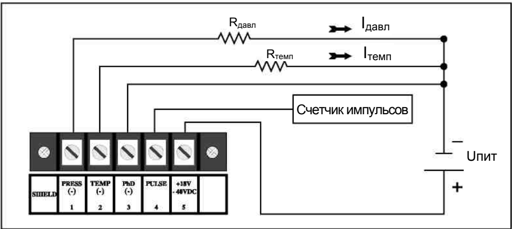
Рис.4.10. Схема подключения импульсного выхода расхода, датчика давления и температуры
