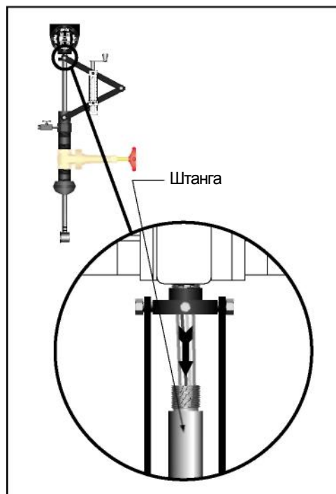
Рис.6.10. Извлечение сенсора V-Bar-600. Отвернуть штангу от монтажного соединения и извлечь штангу вытягиванием со дна расходомера.
