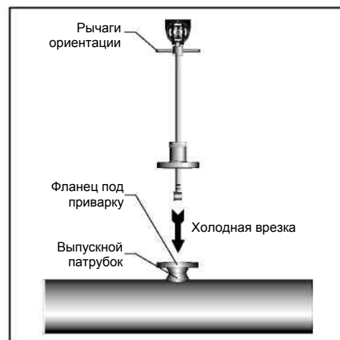
Рис.3.14 Холодная врезка V-Bar-800/80S фланцевого присоединения к выпускному патрубку трубопровода
