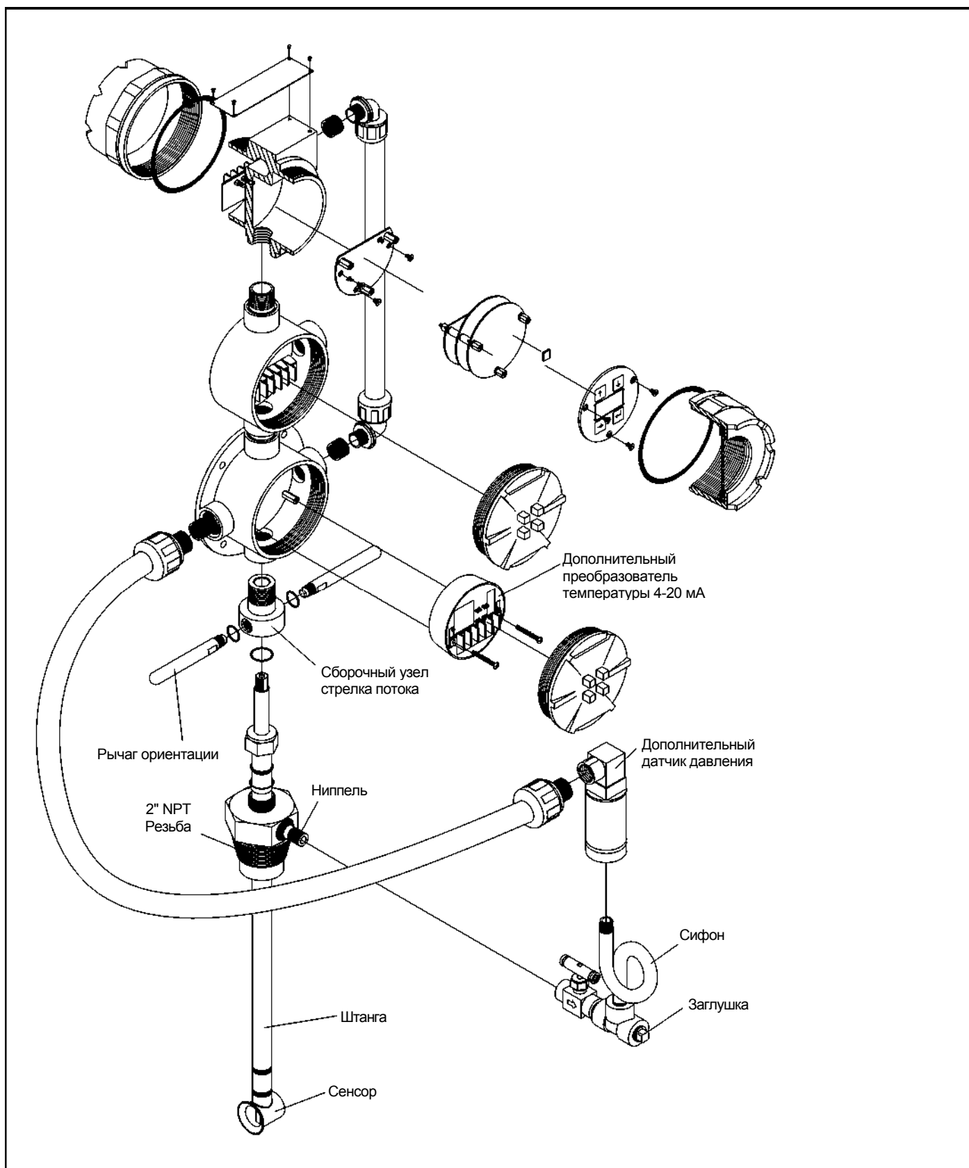
Рис.6.17. V-Bar-700 моноблочное исполнение
