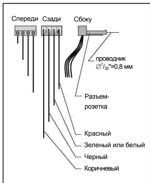
Рис.6.4. Цветная маркировка проводов сенсора.
