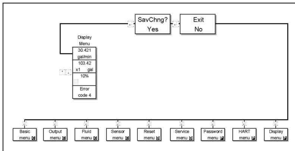
Рис.5.9. Выход из программирования субменю
