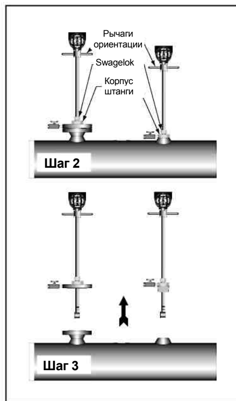
Рис.6.15. Извлечение V-Bar-700
