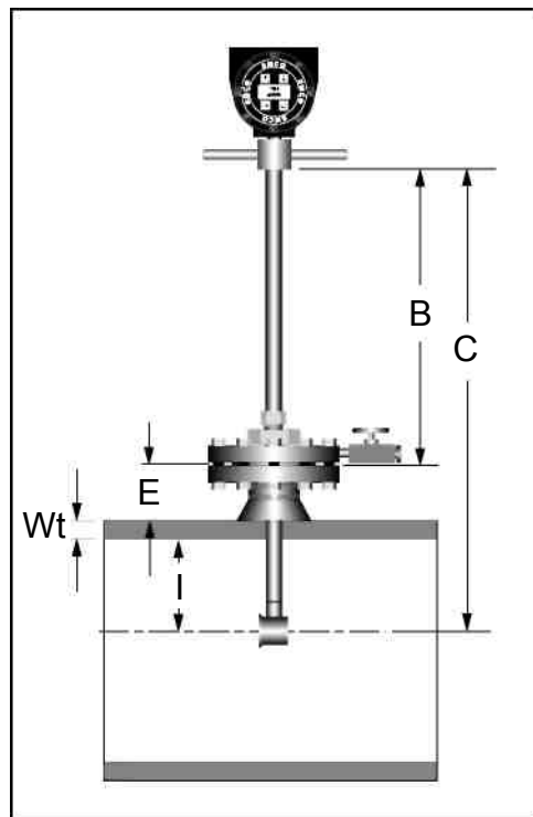
Рис.3.10. Вычисление глубины погружения для V-Bar-700 с фланцевым 2" присоединением
