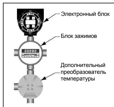
Рис.4.8. Схема подключения
