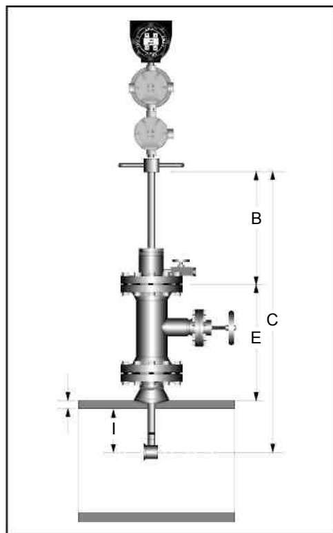
Рис.3.16. Вычисление глубины погружения для фланцевого исполнения V-Bar-800/ 80S
