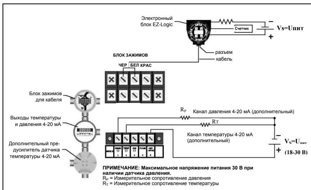
Рис.4.14. Схема подключения датчика давления и термопреобразователя температуры 4-20 мА при раздельном монтаже электронного блока
