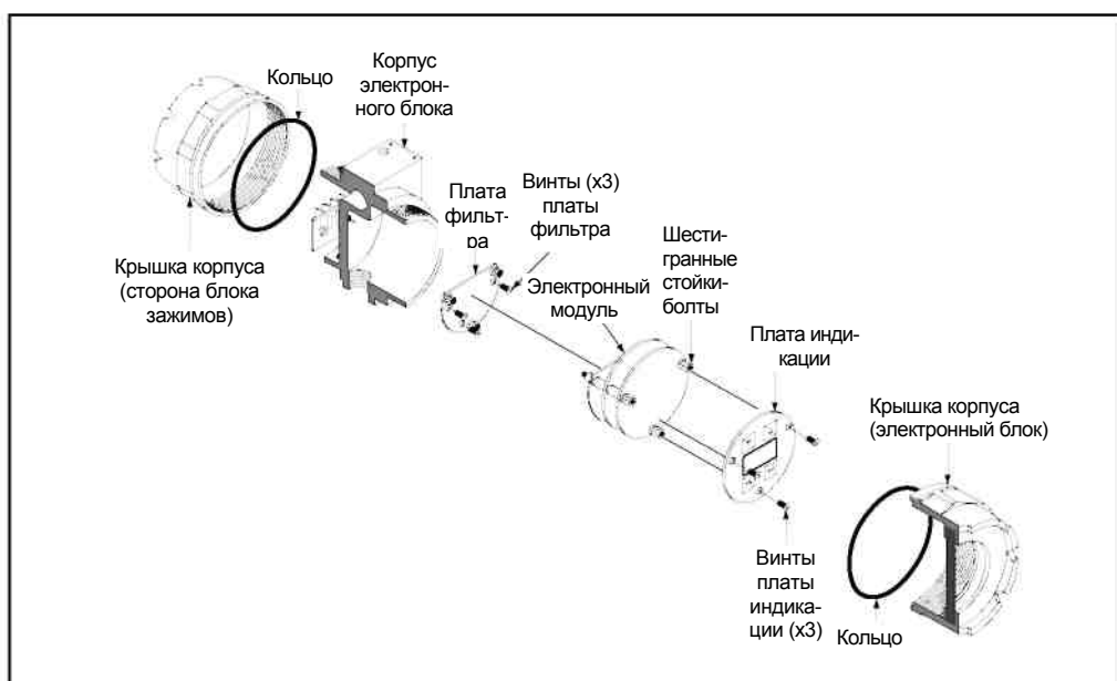
Рис.6.1. Составные части электронного блока
