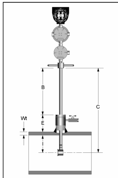
Рис.3.17. Вычисление глубины погружения V-Bar-800/ 80S резьбового присоединения 2" NPT
