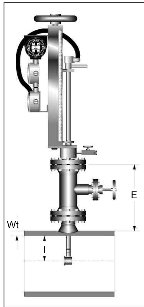
Рис.3.23. Вычисление глубины погружения V-Bar-910/960. Глубина погружения есть сумма измеренных величин I, E и Wt, представленная в дюймах.
