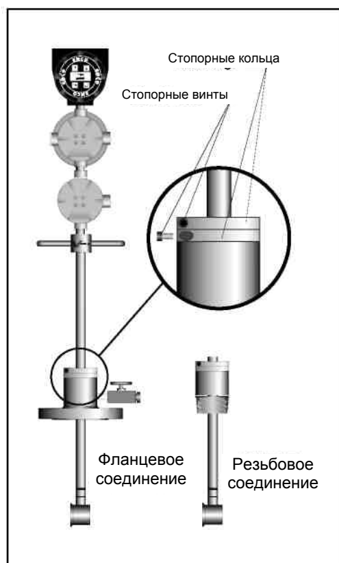
Рис.3.18. Размещение стопорных винтов. Для фиксации штанги в заданном положении, затяните стопорные кольца винтами.
