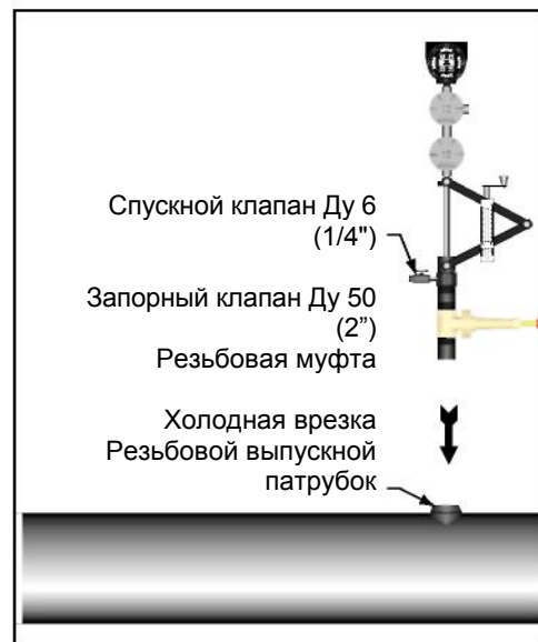
Рис.3.2 Холодная врезка расходомера V-Bar-600/60S
