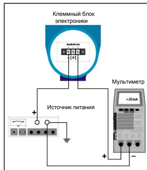
Рис.5.8. Схема соединений для калибровки выхода 4-20 мА
