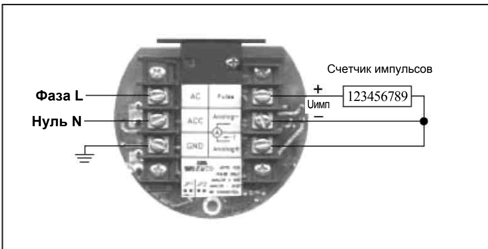
Рис.4.12. Схема подключения с импульсным выходом (установлена перемычка JP2)
