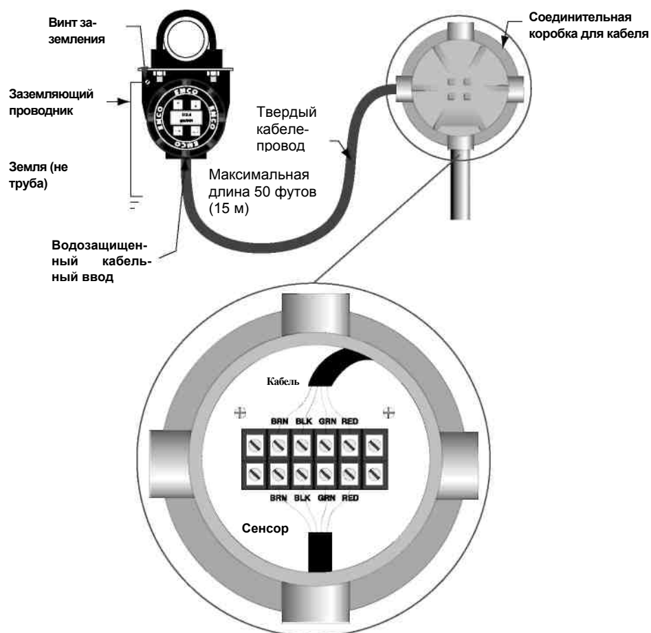
Рис.4.13. Схема подключения для раздельного исполнения электронного блока
