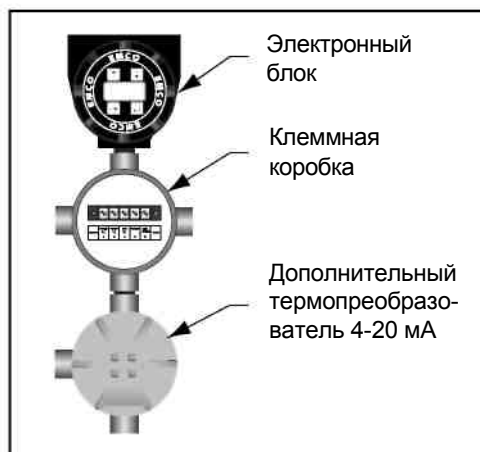
Рис.6.21. Расположение клеммной коробки
