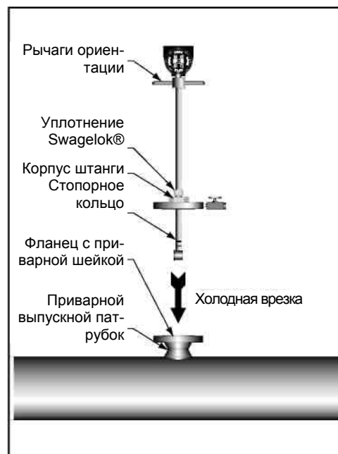
Рис.3.8. Установка V-Bar-700 с фланцевым присоединением к трубопроводу
