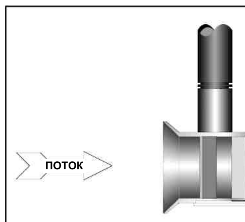
Рис.6.31. Вход вихревой головки сенсора. При сборке штанги стрелка направления потока и вход вихревой головки сенсора (раструб) направлены навстречу друг другу.
