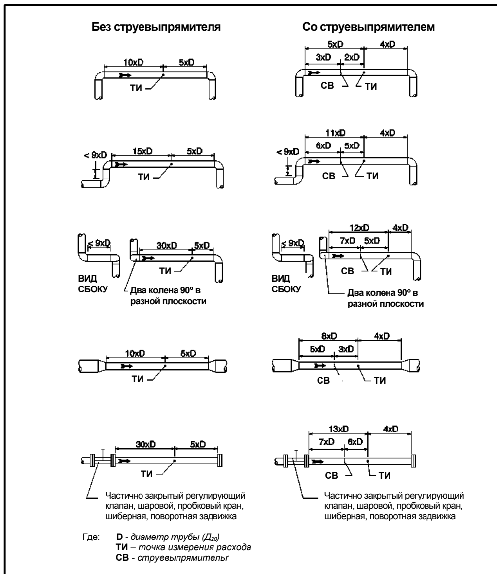
Рис.2-1. Требования к прямым участкам. Полностью открытый клапан соответствует одиночному колену
