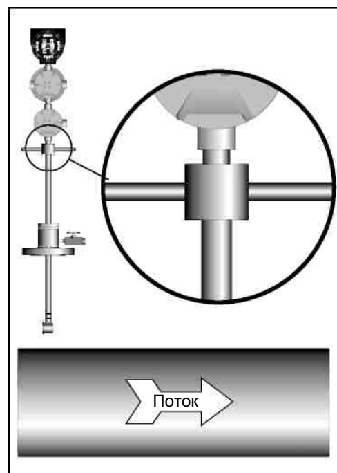
Рис.3.20. Ориентация расходомера V-Bar-800/80S. Сориентируйте расходомер так, чтобы рычаги ориентации были параллельны оси трубы, а стрелка на корпусе совпадала с направлением потока среды.
