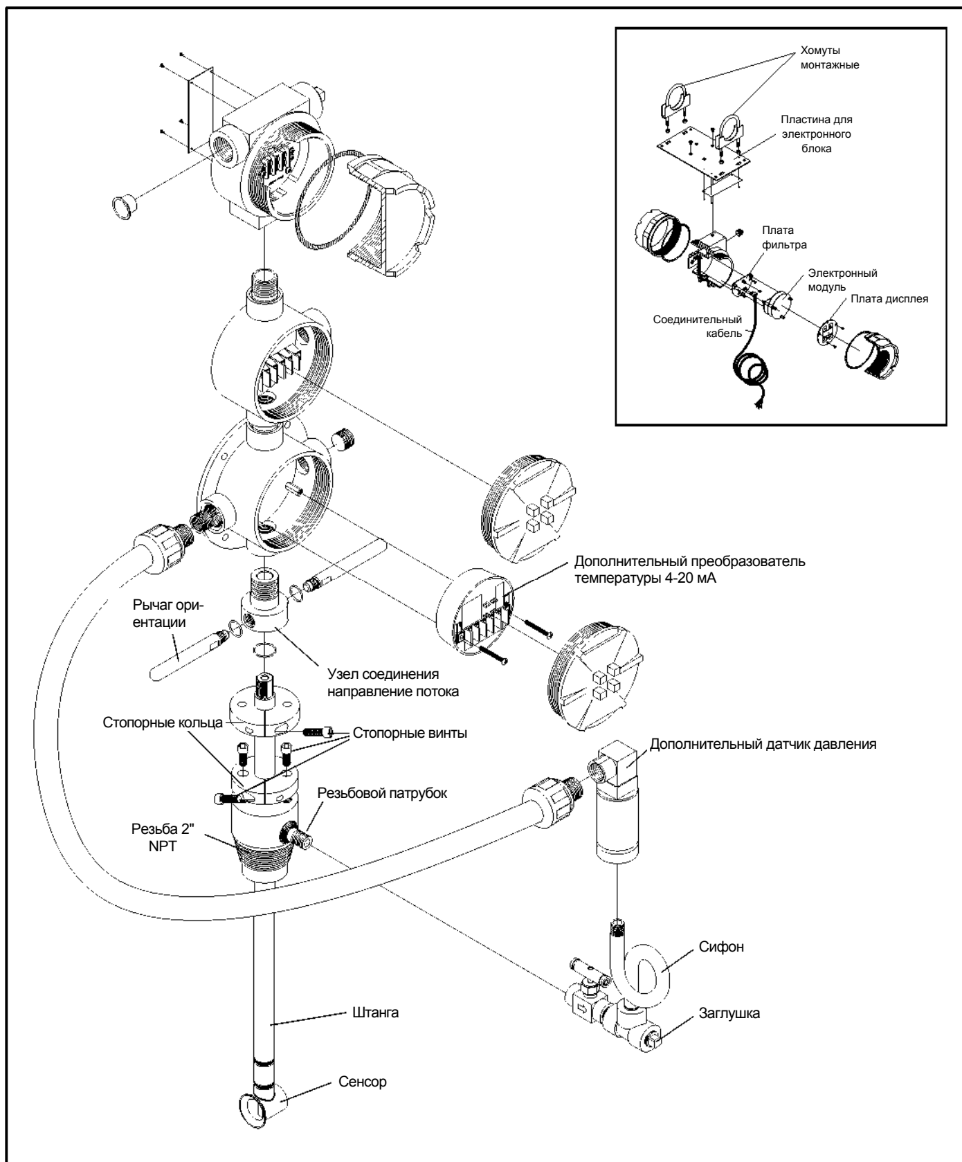
Рис.6-26. Расходомер V-Bar-800/80S раз- дельный монтаж
