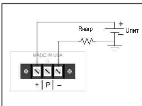
Рис.4.5. Схема подключения для аналогового выхода (нет перемычек или установлена JP1)
