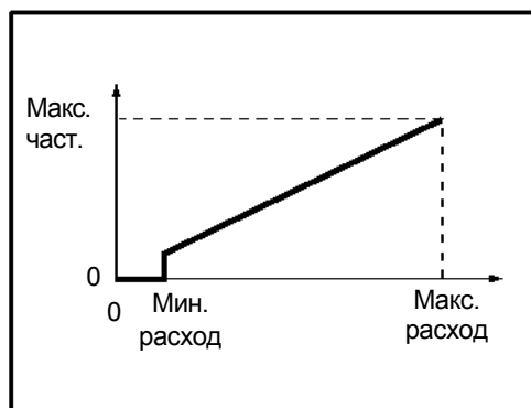
Рис.5.6. Линейный масштабируемый частотный выход
