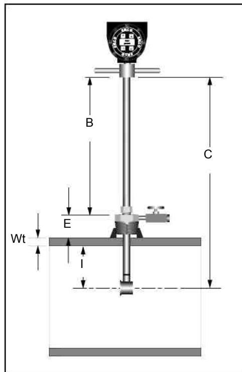
Рис.3.9. Вычисление глубины погружения для V-Bar-700 с резьбовым 2" присоединением
