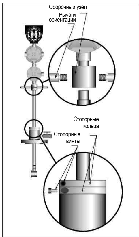
Рис.6.20. Извлечение сенсора V-Bar-800. Отвернуть штангу от монтажного соединения и извлечь штангу вытягиванием со дна расходомера
