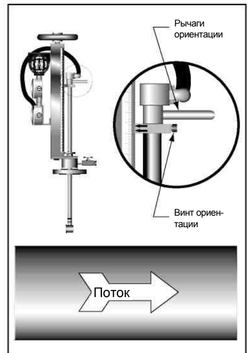
Рис.3.26. Ориентация расходомера V-Bar-910/960. Сориентируйте расходомер так, чтобы рычаги ориентации были параллельны оси трубопровода, а стрелка на корпусе была по направлению потока в трубе.
