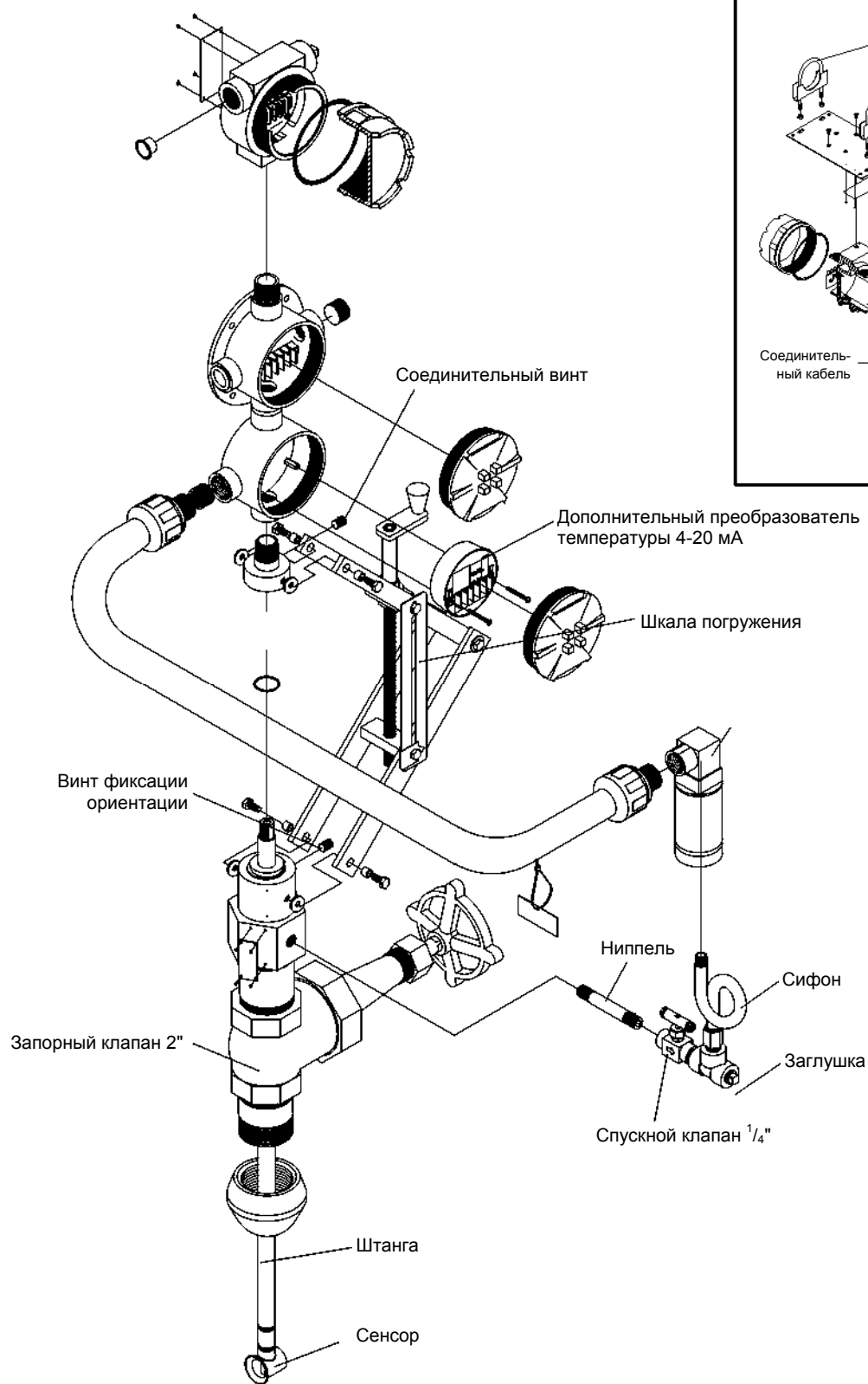
Рис.6.14. Сборочный чертеж V-Bar-600/60S раздельного исполнения
