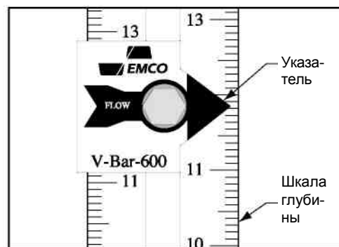
Рис 3.3. Отсчет по шкале V-Bar-600/60S. Отсчет по шкале это цифра на которую указывает курсор. Отсчет по шкале равен глубине погружения сенсора.
