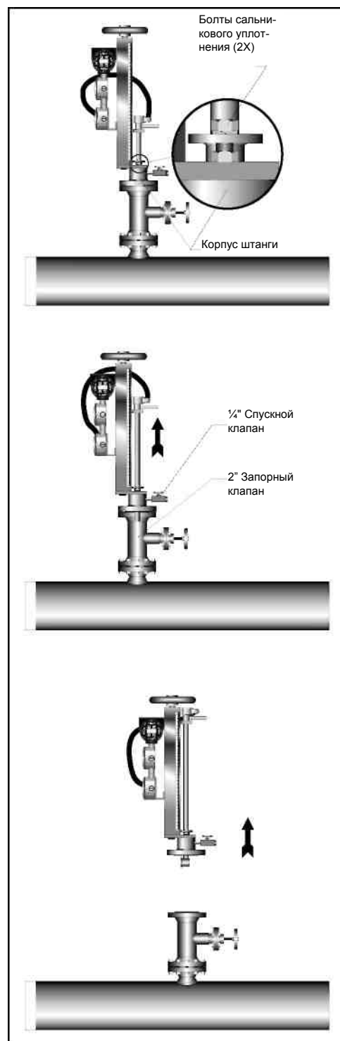
Рис.6.27. Извлечение V-Bar-910/960
