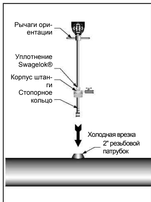
Рис.3.7. Установка V-Bar-700 с 2" NPT резьбовым присоединением к трубопроводу
