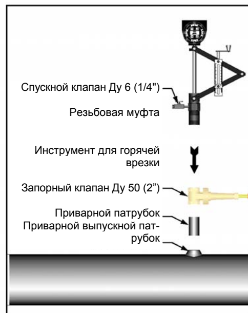
Рис.3.1 Горячая врезка расходомера V-Bar-600/60S
