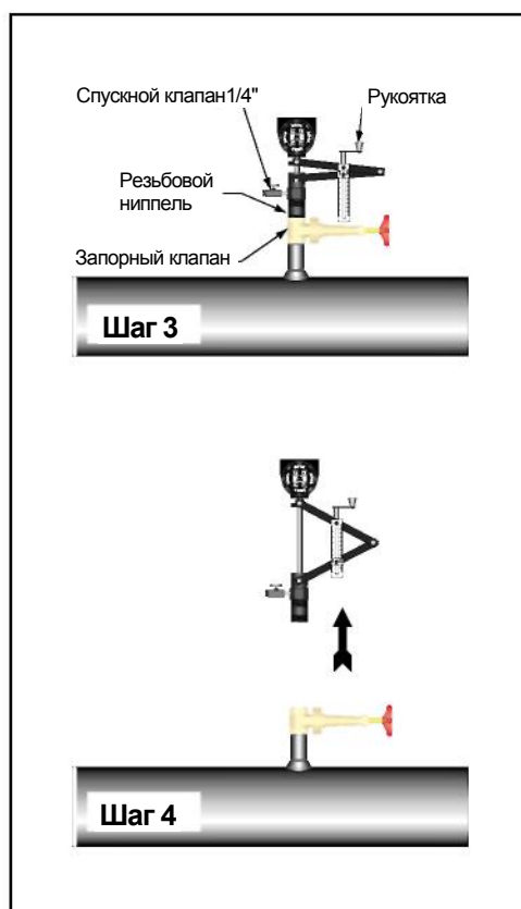
Рис.6.6. Извлечение V-Bar-600/60S
