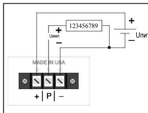
Рис.4.6. Схема подключения импульсного выхода (установлена JP2)
