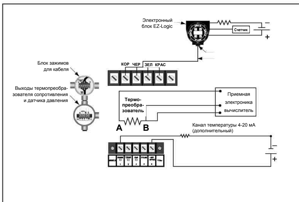
Рис.4.15. Схема подключения датчика давления и термопреобразователя сопротивления при раздельном монтаже электронного блока
