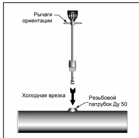
Рис.3.15 Холодная врезка V-Bar-800/80S резьбового присоединения к выпускному патрубку трубопровода
