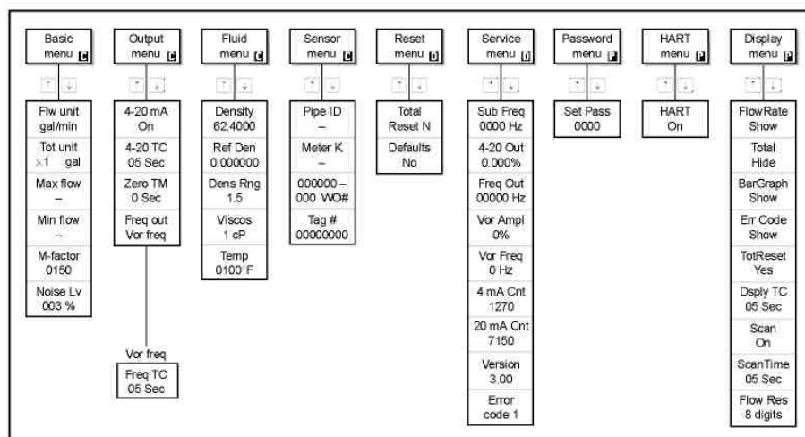
Рис.5.7. Установки по умолчанию
