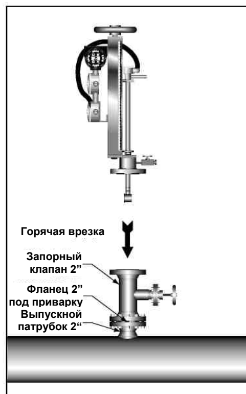
Рис.3.21. Горячая врезка V-Bar-910/960
