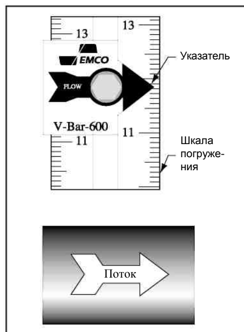
Рис.3.5. Ориентация по потоку V-Bar-600/60S. Сориентируйте расходомер так, чтобы направление потока совпадало со стрелкой на шкале.
