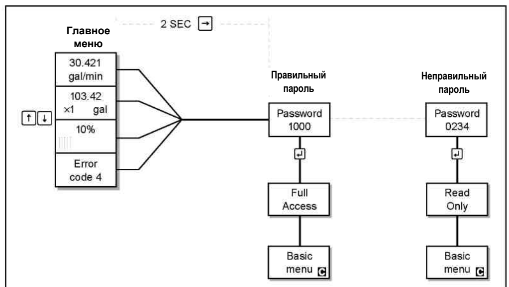
Рич.5.4. Пароль доступа к субменю
