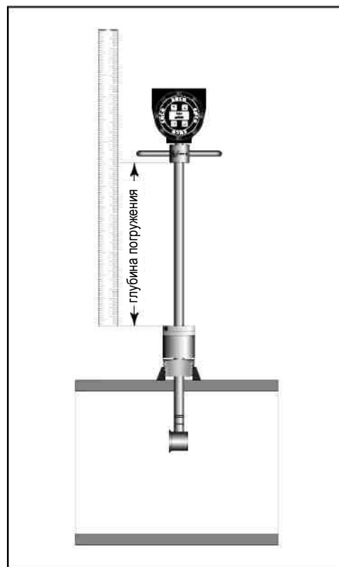
Рис.3.19. Окончательное позиционирование V-Bar-800/80S. Вручную введите штангу в трубу пока требуемая глубина погружения не будет обеспечена
