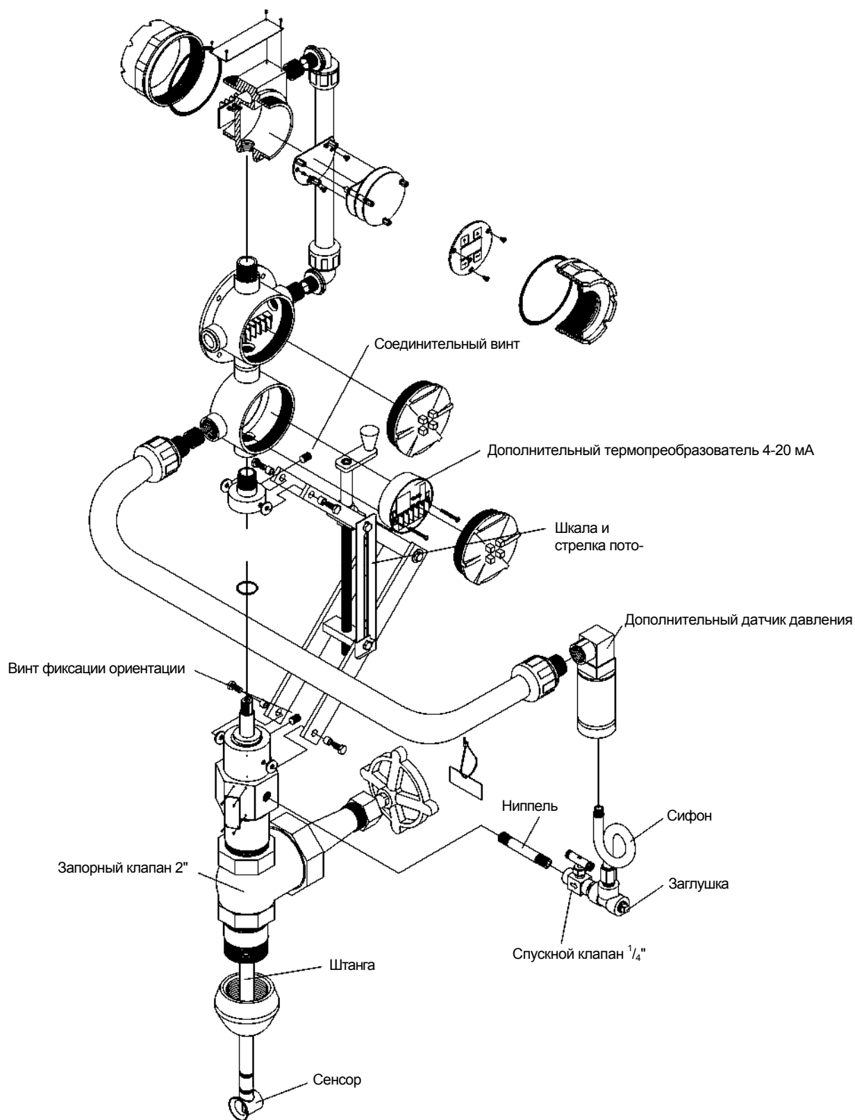
Рис.6.13. V-Bar-600/60S моноблочного исполнения
