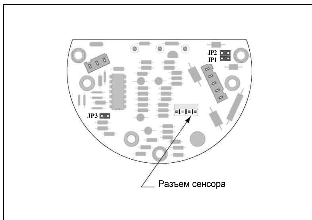
Рис.6.3. Размещение разъема сенсора на плате фильтра
