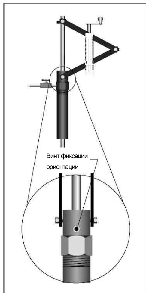
Рис.6.5. Разположение винта фиксации ориентации. Чтобы освободить штангу ослабьте винт фиксации ориентации.
