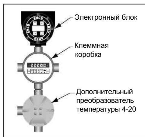
Рис.6.8. Расположение клеммной коробки
