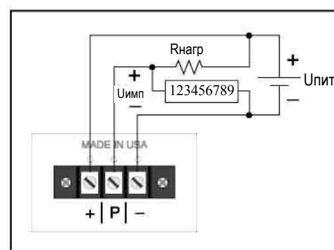
Рис.4.7. Схема подключения для импульсного выхода (нет перемычек)
