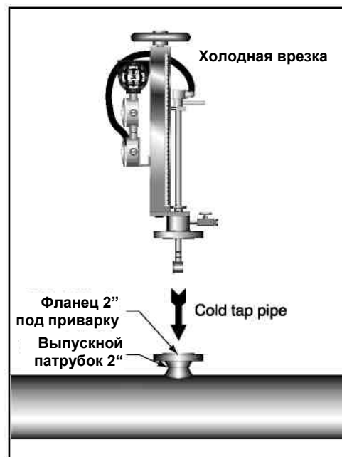
Рис.3.22. Холодная врезка V-Bar-910/960
